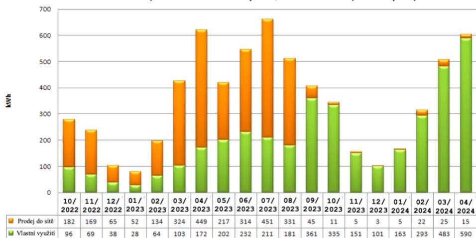
Využití elektřiny z FVE Senior Centrum Starý Mateřov 400 - reálná data provozu mikrozdroje 5 kWp
