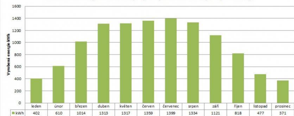
Elektrárna o výkonu 10kWp - předpoklad roční výroby elektřiny
